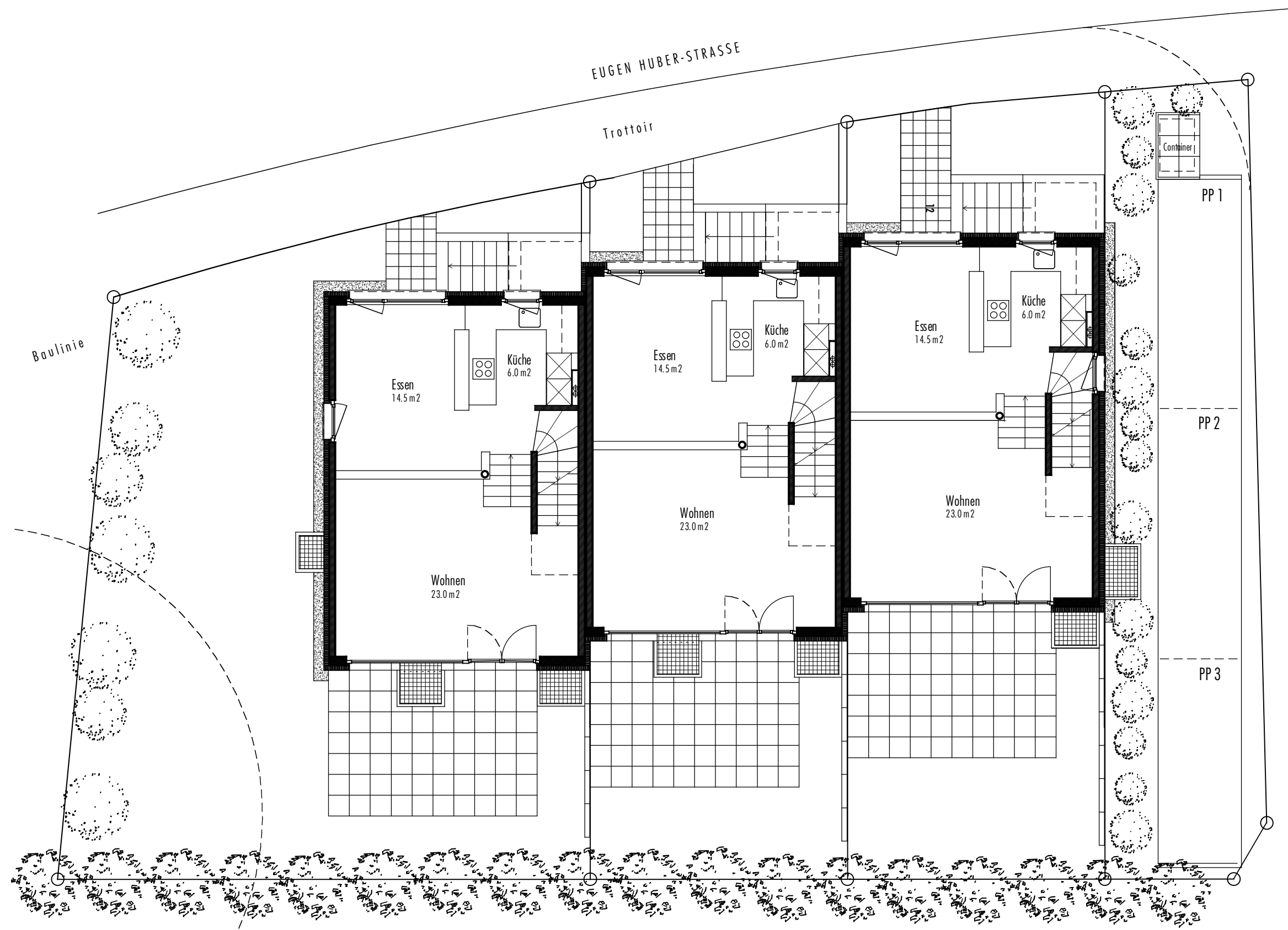
ERDGESCHOSS
